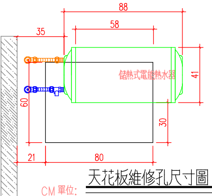
儲熱式電能熱水器安裝施工示意圖
